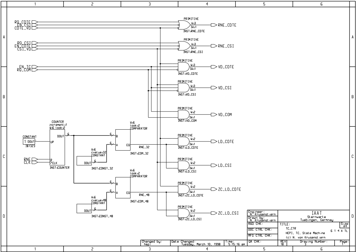
Abbildung 42: Das Schematic des Sub-Moduls TC_CTR
