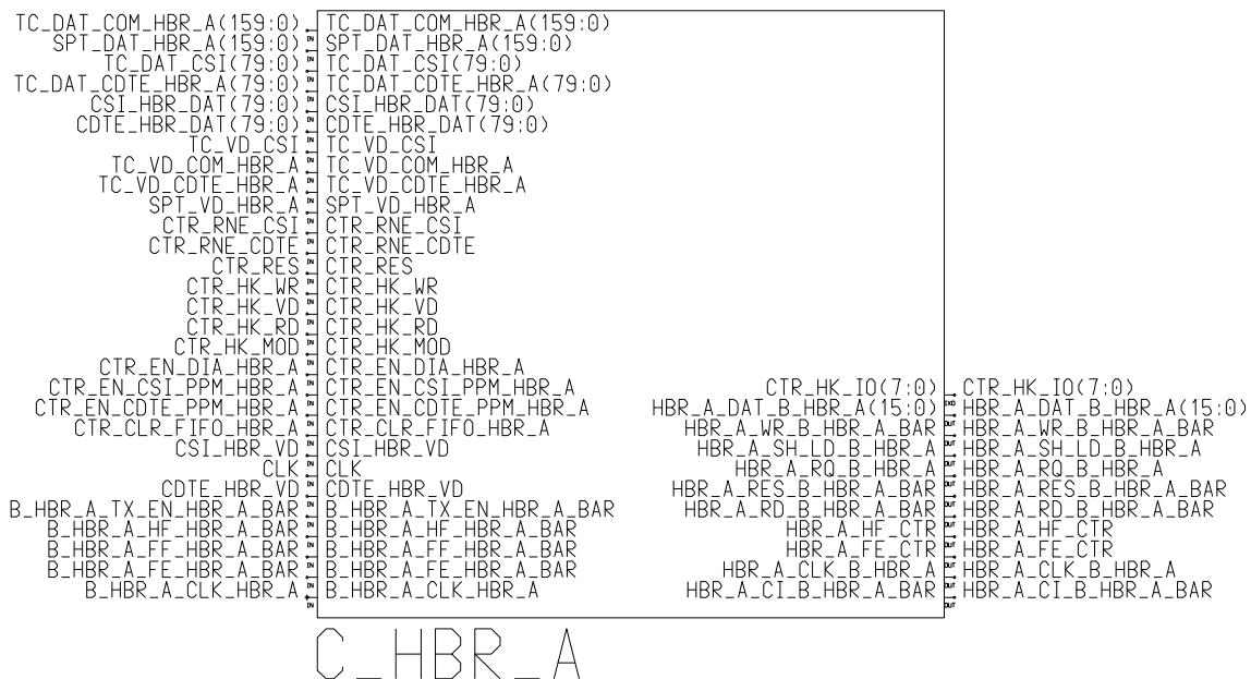
Abbildung 23: Das Symbol der Schnittstelle A zur DPE
