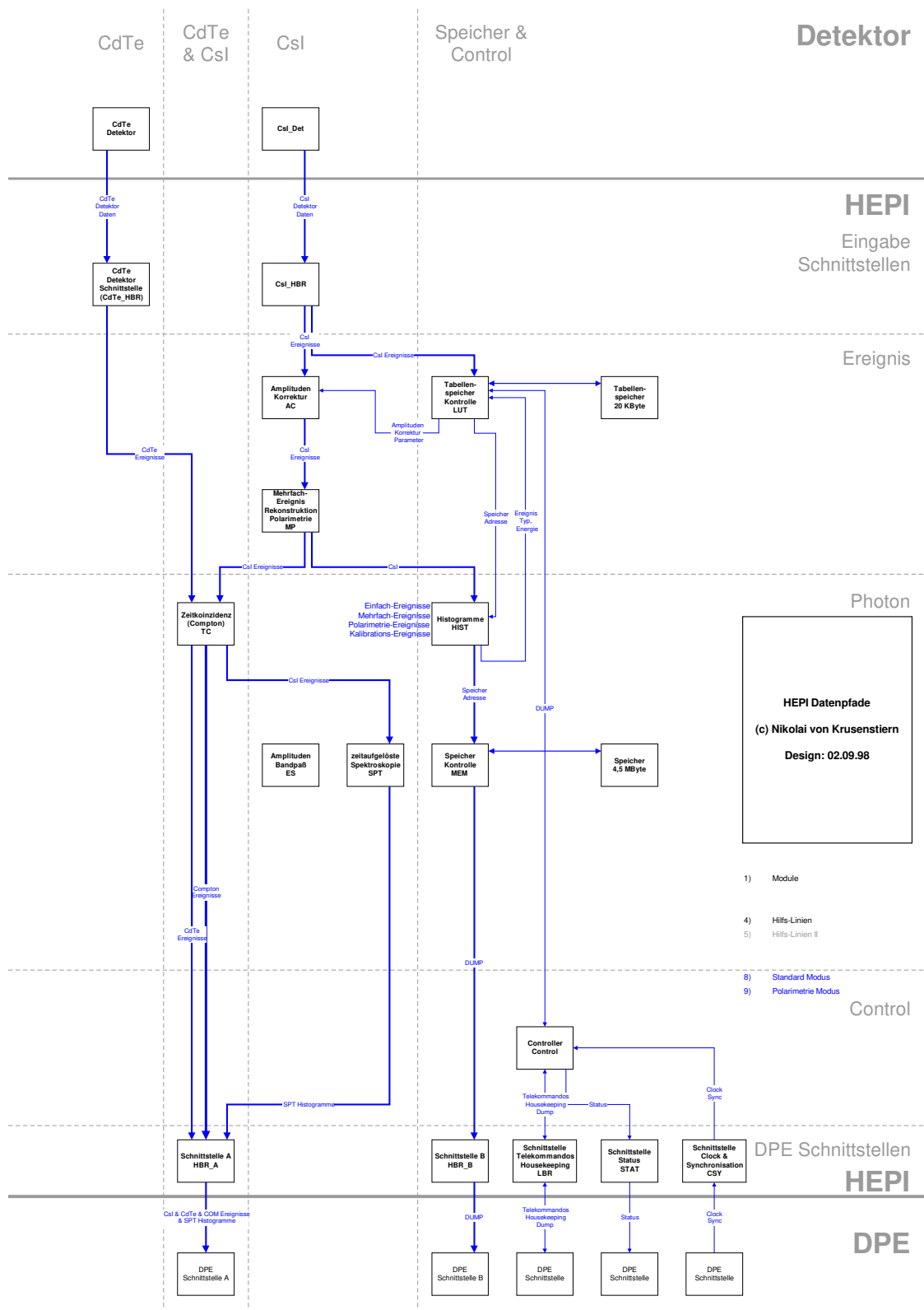
Abbildung 53: Der Standard Pointing und Standard Polarimetry Modus
