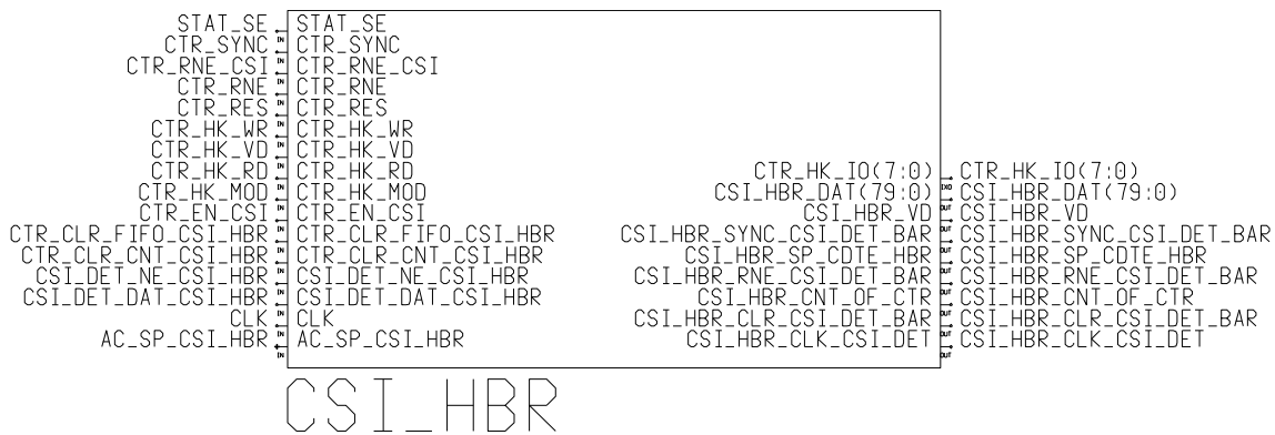
Abbildung 22: Das Symbol der Schnittstelle zum Cäsium-Jodid-Detektor
