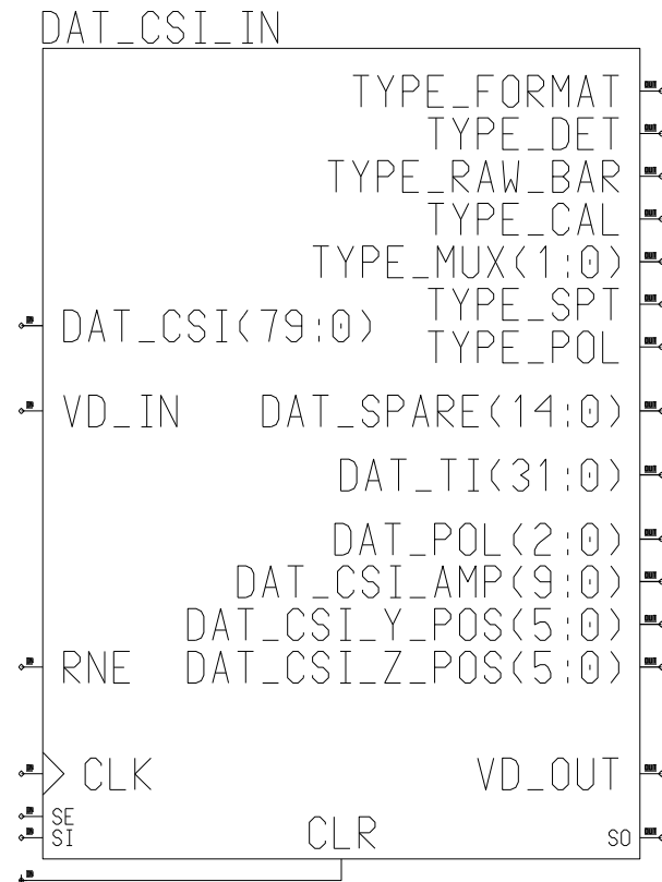
Abbildung 17: Die Eingabe-Schnittstelle für Cäsium-Jodid-Ereignisse
