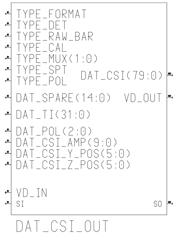
Abbildung 18: Die Ausgabe-Schnittstelle für Cäsium-Jodid-Ereignisse
