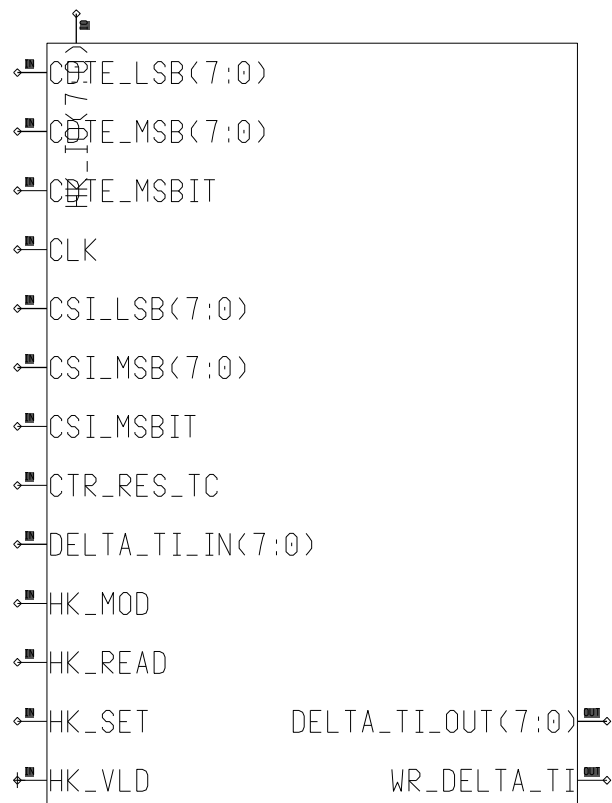
Abbildung 20: Die Ein- und Ausgabe-Schnittstelle für Housekeeping-Daten
