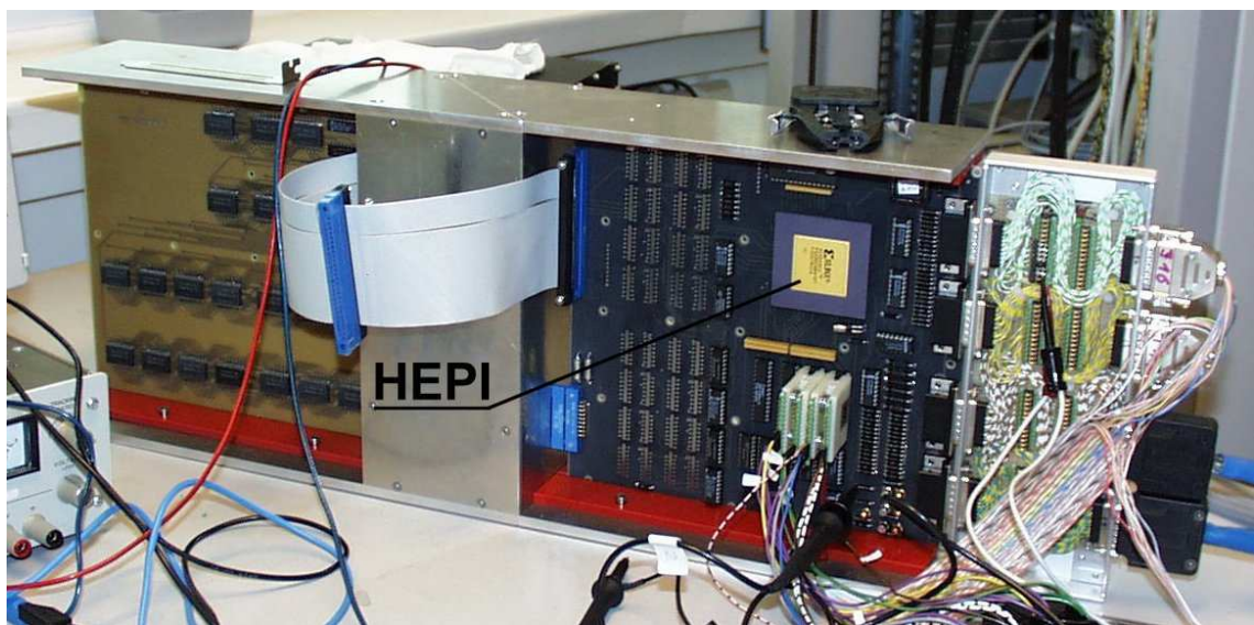
Abbildung 1: Ein Foto der HEPI-Platine und der HEPI (FPGA) 7
