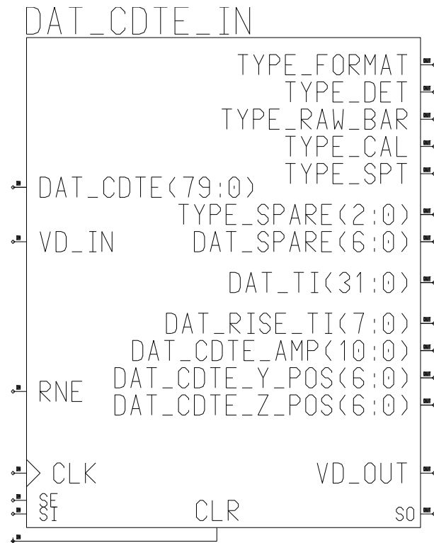
Abbildung 15: Die Eingabe-Schnittstelle für Cadmium-Tellurid-Ereignisse
