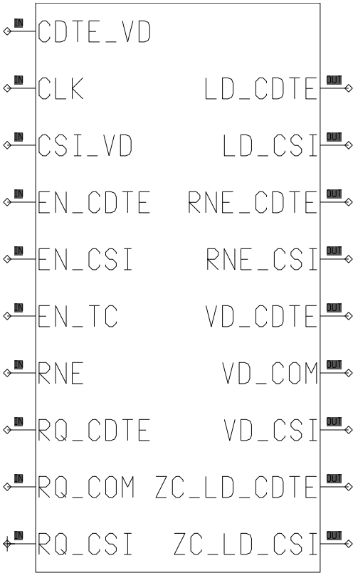
Abbildung 41: Das Symbol des Sub-Moduls TC_CTR
