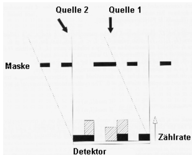
Abbildung 7: Die kodierte Aperturmaske, zweidimensional 25
