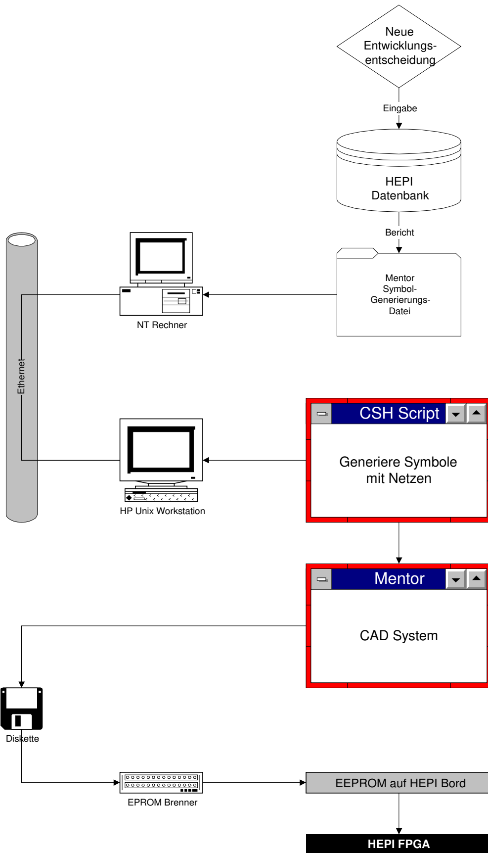
Abbildung 11: Der Designfluß des Entwicklungskonzeptes
