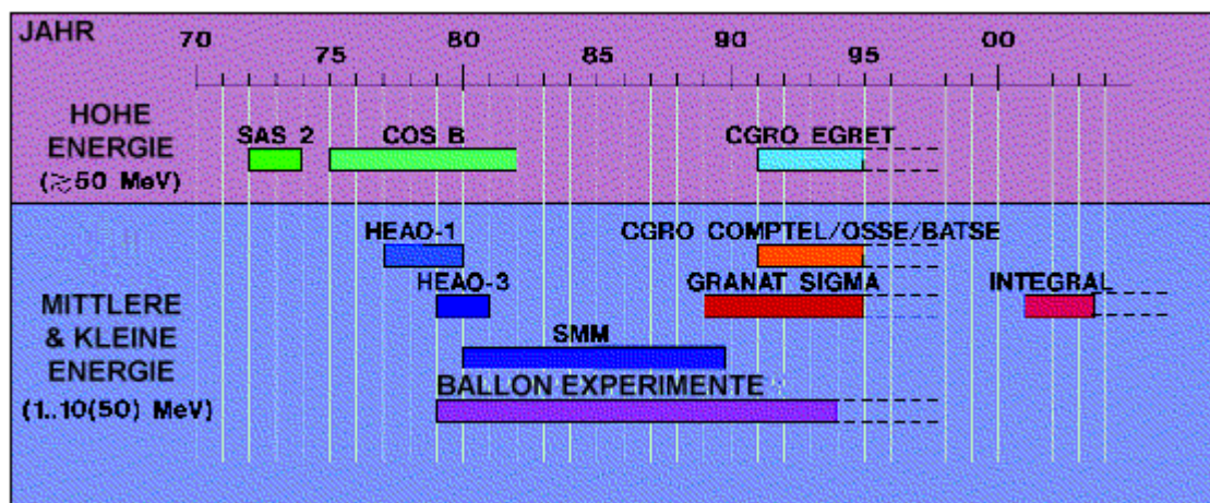
Abbildung 2: Ein Überblick über einige astronomische Gammastrahlen-Experimente 15
