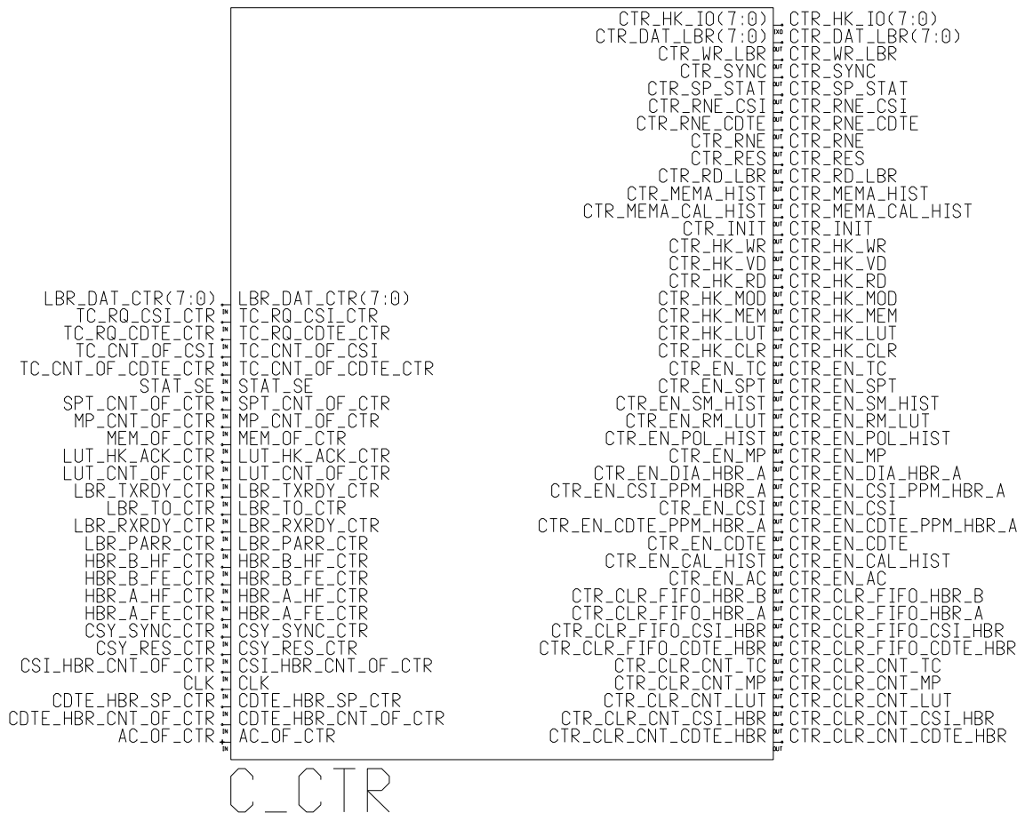
Abbildung 30: Das Symbol des Controllers
