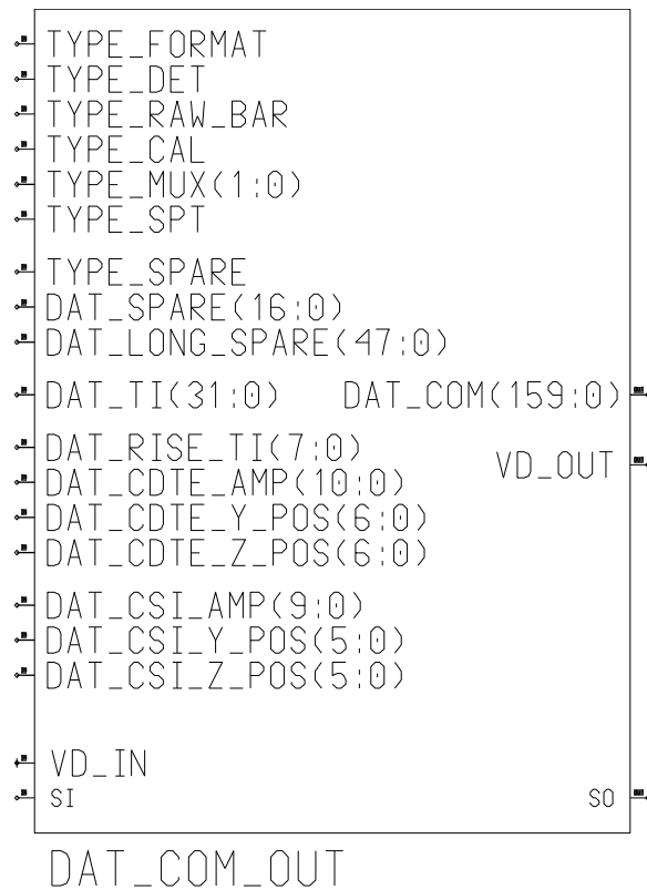
Abbildung 19: Die Ausgabe-Schnittstelle für Compton-Ereignisse
