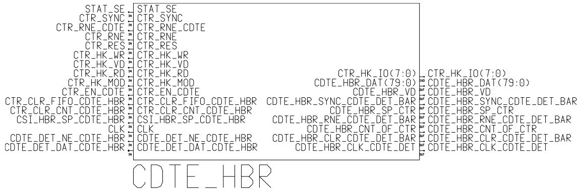
Abbildung 21: Das Symbol der Schnittstelle zum Cadmium-Tellurid-Detektor
