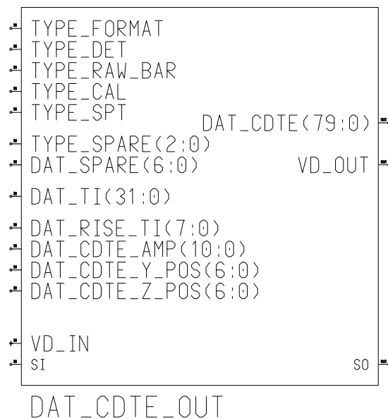
Abbildung 16: Die Ausgabe-Schnittstelle für Cadmium-Tellurid-Ereignisse
